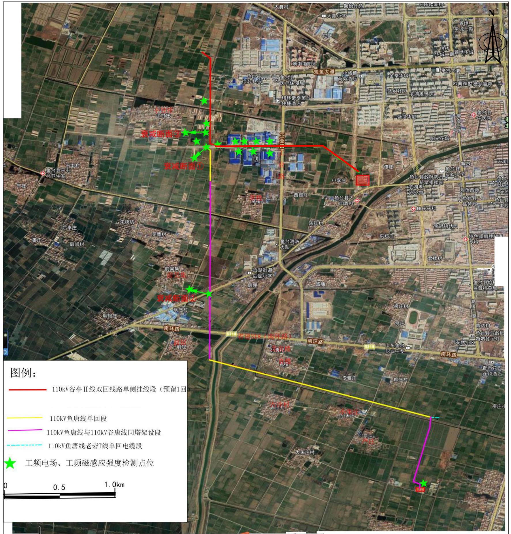
图 7-1 本项目工频电场、工频磁感应强度检测布点图
